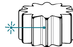
Измерение шага цилиндрических зубчатых колёс
